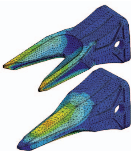
Mit modernster 3D-CAD- Software konstruiert und auf Belastung geprüft: die neuen VIP-Zähne der maXforce-Serie.
